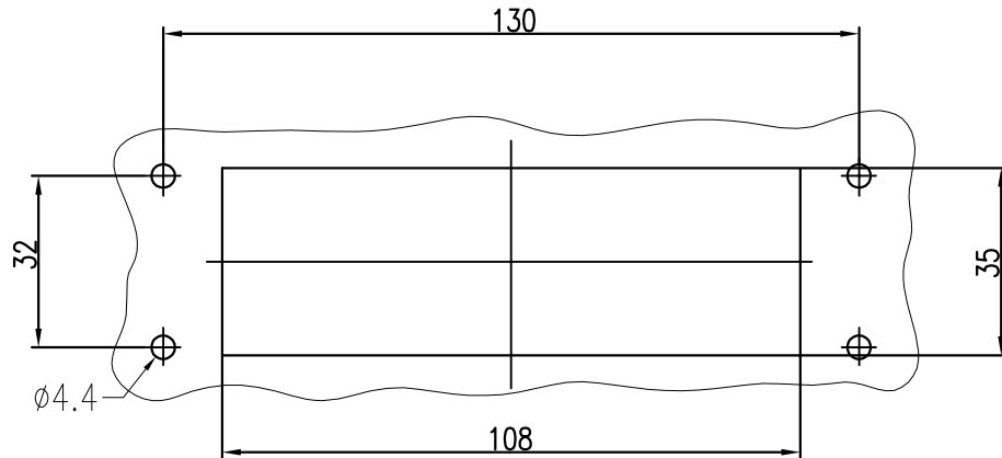
面板开孔图
